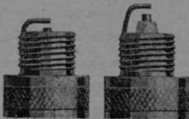
Aislador de punta más larga que en bujías ordinarias
